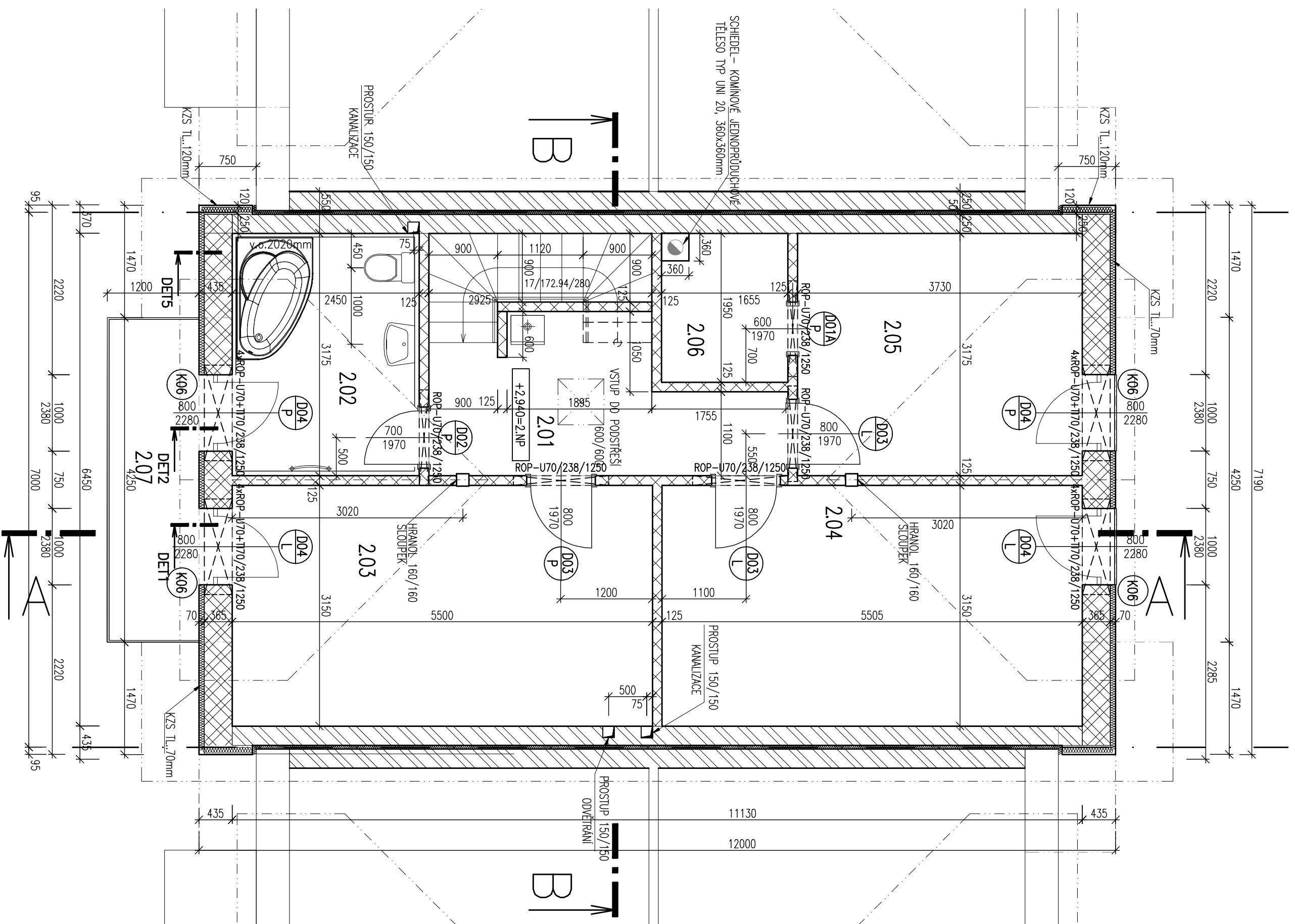
TABULKA MÍSTNOSTI
